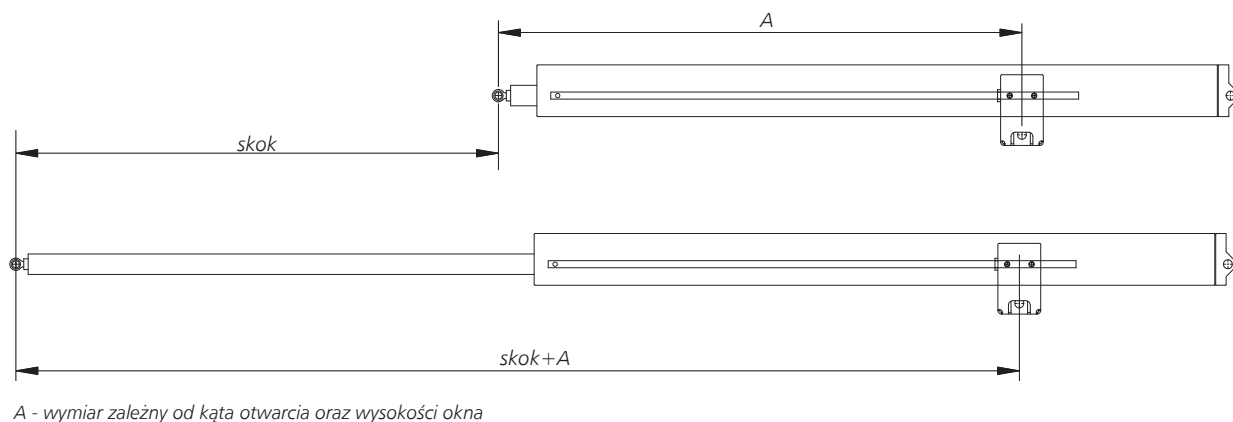
Rys. 102 Wymiary siłownika wrzecionowego typ G z przesuniętym punktem obrotu
