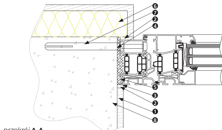
przekrój A-A
