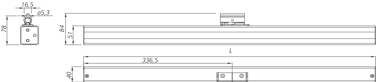
Rys. 115 Wymiary siłownika elektrycznego łańcuchowego HCVA, wymiary [mm]
