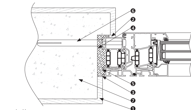
przekrój A-A
